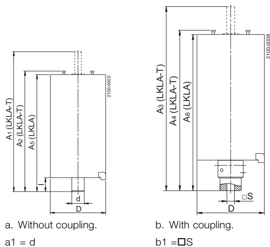
Fig. 2. Dimensions - actuator
